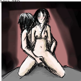
Monoceros01 2006 Elisa 2005
