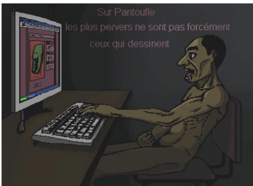
Monoceros01 2006 Elisa 2005
