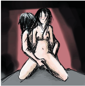
Monoceros01 2006 Elisa 2005
